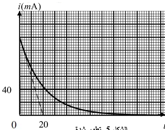
الشكل 5. تطور شدة التيار بدلالة الزمن
