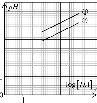
الشكل 5. تطور الـ pH بدلالة -\log[HA]_{eq}
