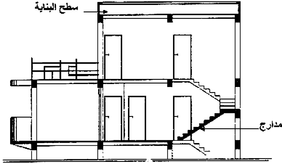
جزء من مقطع عمودي للبناية الإدارية .
